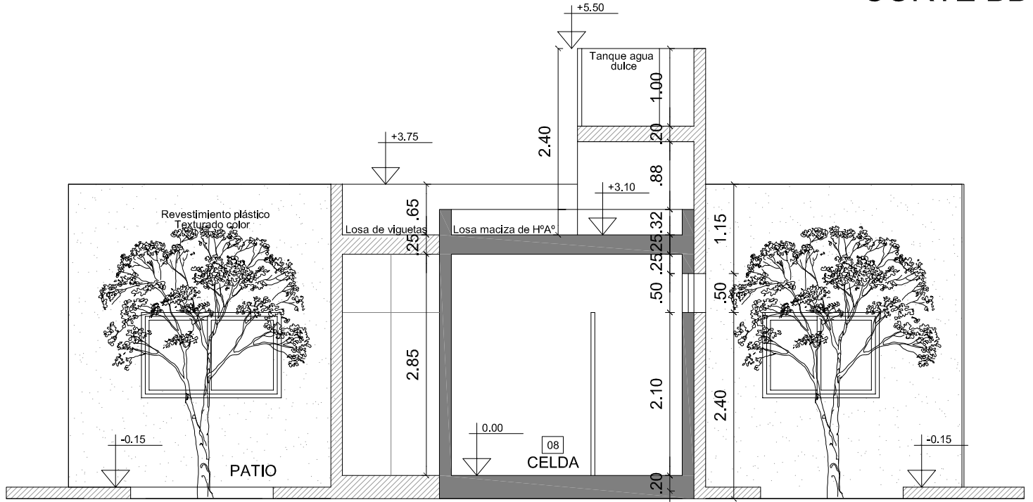
CORTE CC
