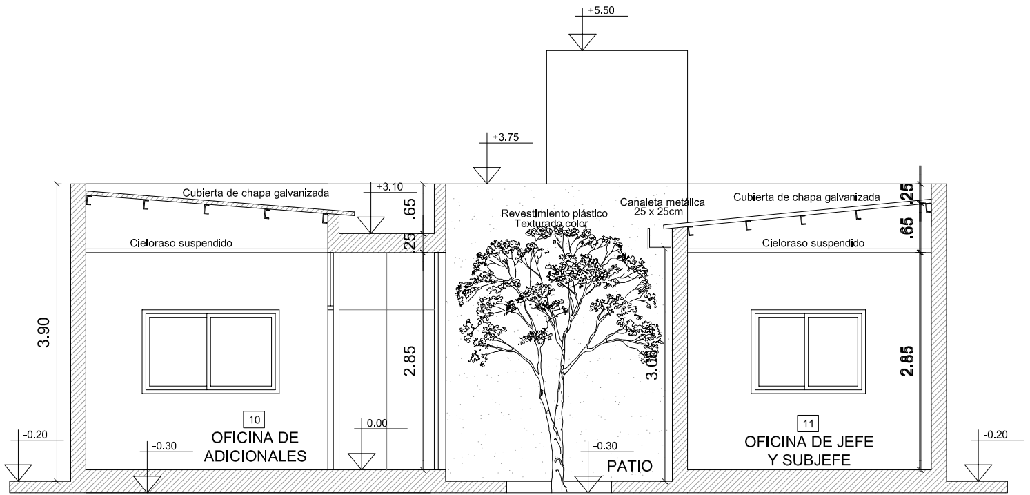
CORTE BB
