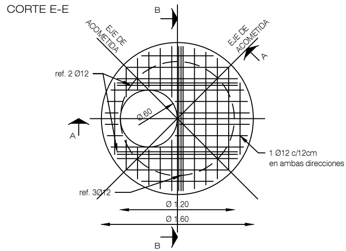
DETALLE DE ARMADURAS
